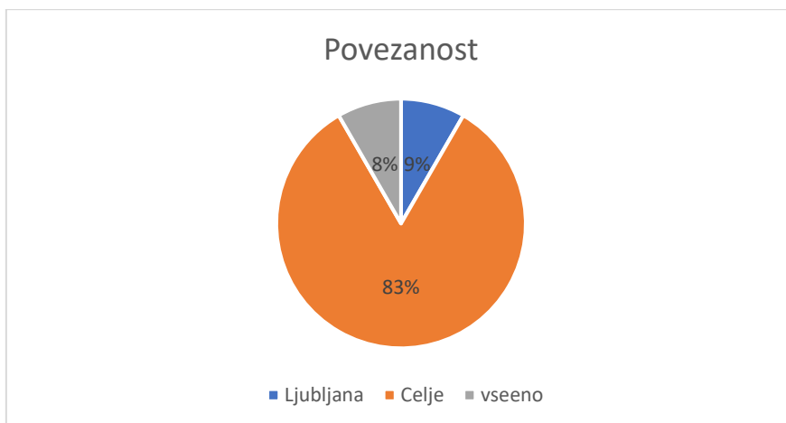
Graf 4: Povezanost
