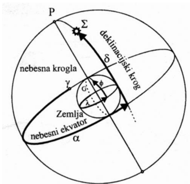
Slika 3: Ekvatorialni koordinatni sistem
