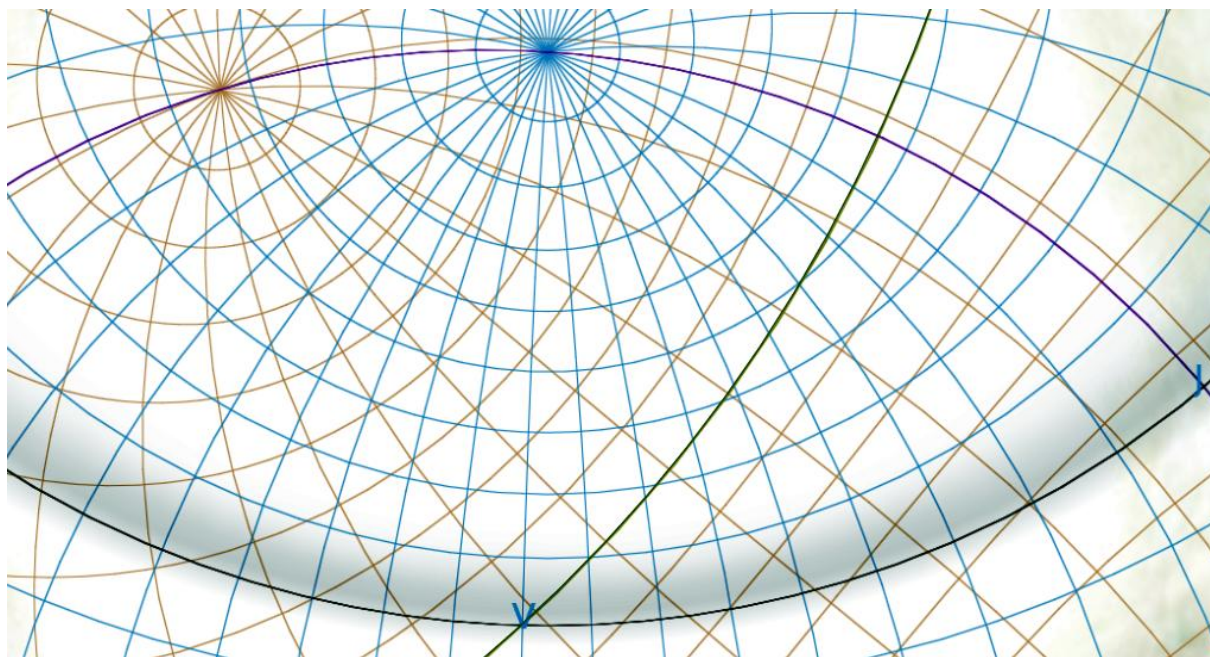
Slika 2: Nebesna koordinatna sistema
